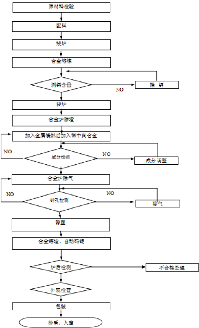
图 2.3.1：铝合金锭生产加工过程
